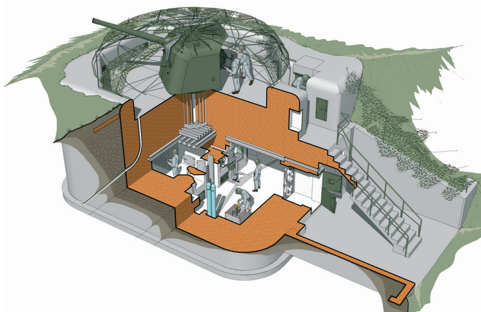
Widok z przekrojem stanowiska ogniowego
