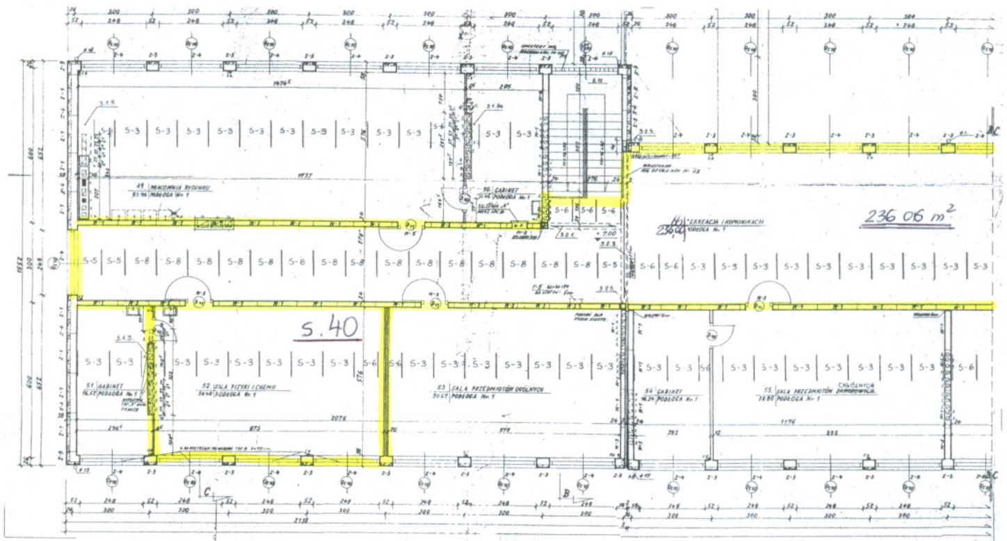
RZUT II PIĘTRA - B
