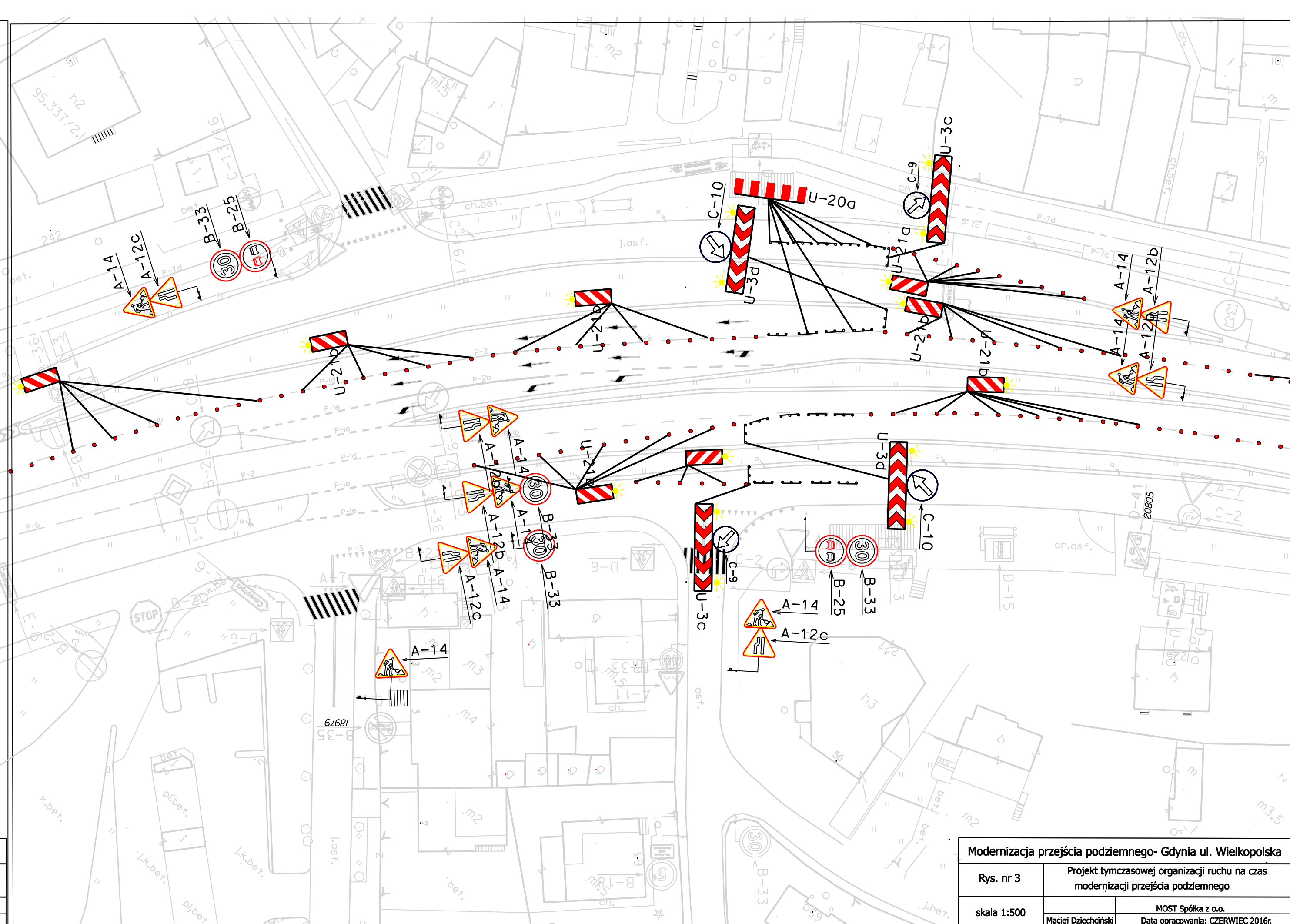
Modernizacja przejścia podziemnego- Gdynia ul. Wielkopolska Rys. nr 2 Projekt tymczasowej organizacji ruchu na czas modernizacji przejścia podziemnego skala 1:500 Miejsc. Dwiechfolki Data opracowania: CZERWIEC 2016r.
