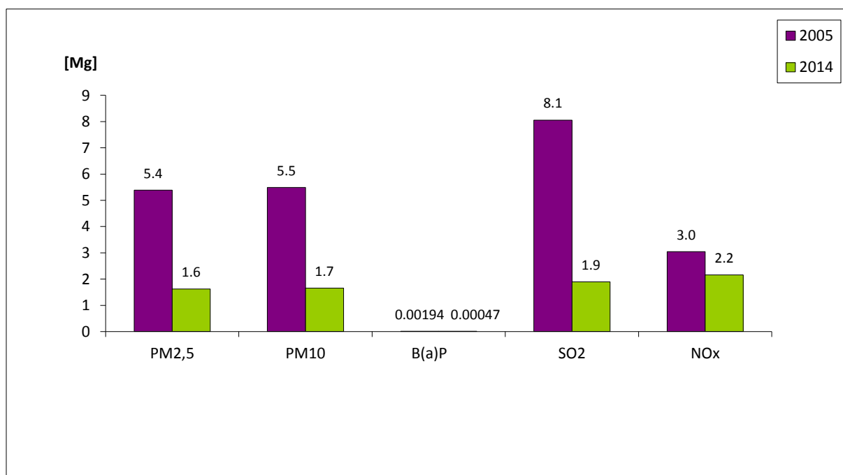
Rysunek 7. Emisja pozostałych zanieczyszczeń w 2005r. i 2014r. - obiekty użyteczności publicznej.
