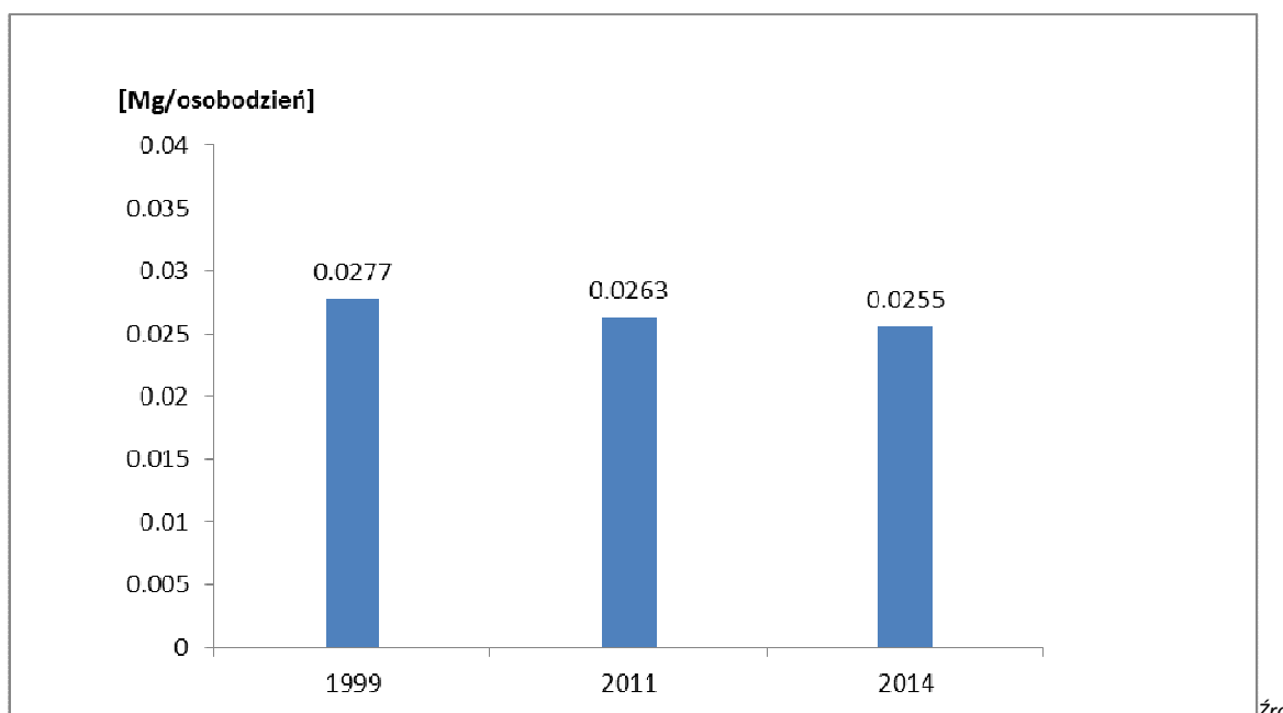
Rysunek 26. Emisja CO 2 na jeden osobdzień (mieszkańcy oraz turyści) z pominięciem przemysłu.
