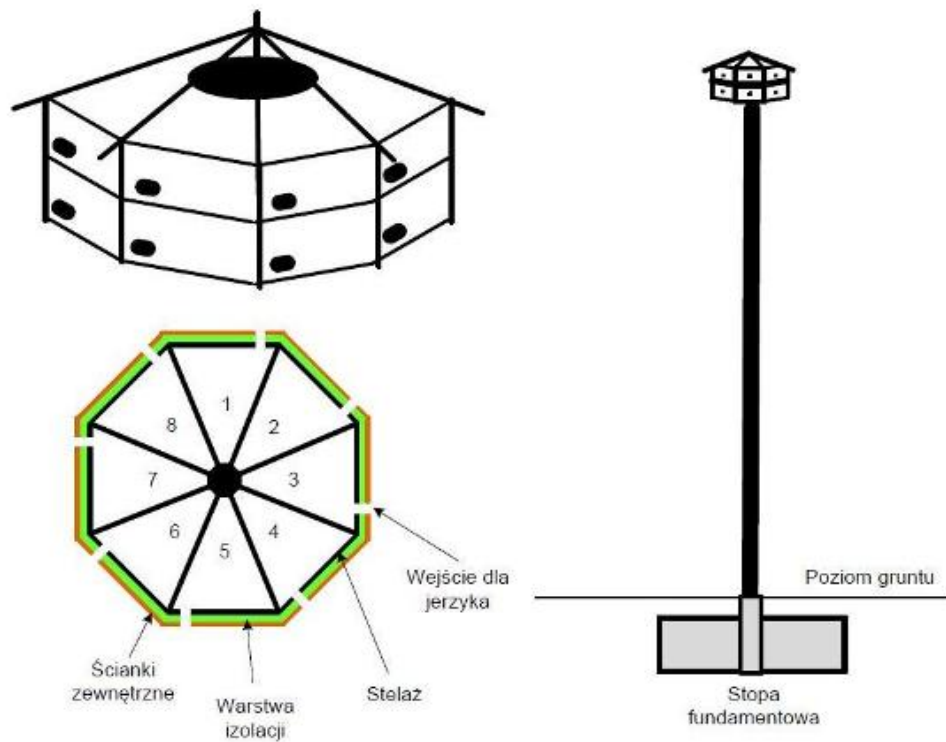
Rys. 1. Konstrukcja wieży
