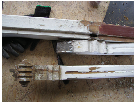
4, 5, 6. Dekoracyjny detal okien d. Zajazdu Adlera przy ul. Orłowskiej 8 w trakcie prac konserwatorskich. Prace konserwatorskie polegały m.in. na usunięciu powłok malarskich poprzez podgrzewanie i zdejmowanie szpachelką grubych warstw farb, następnie uzupełnianie były ubytki w drewnie, elementy były szlifowane, malowane i ponownie szklone. Część zniszczonych elementów trzeba było zrekonstruować, ale okna pochodzą z XIX w. Prace wykonano w ramach kompleksowej rewitalizacji budynku trwającej w latach 2011-2013.
