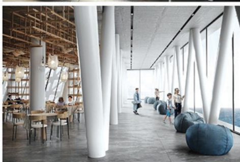
Konstrukcja budynku Muzeum Żeglarstwa jest zaprojektowana jako żelbetowa, monolityczna konstrukcja słupowo-płytowa z fundamentem na monolitycznej płycie fundamentowej na prefabrykowanych palach. Całkowita wysokość budynku wynosi 87 metrów. // fot. mat. prasowe
